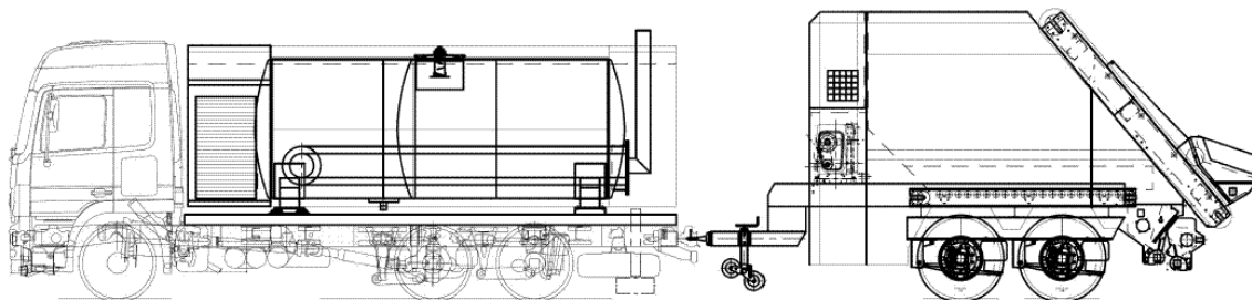
Rys. 1. Schemat kombajnu drogowego do powierzchniowego utwalania nawierzchni
